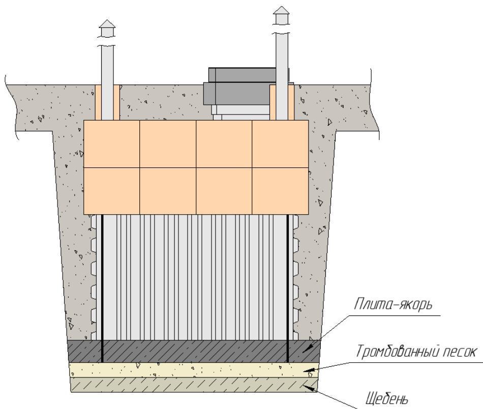
Схема монтажа погреба Т1500 с нижним якорением
