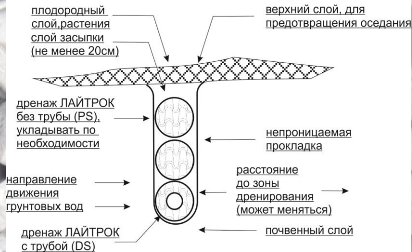
дренаж для стока поверхностных вод
